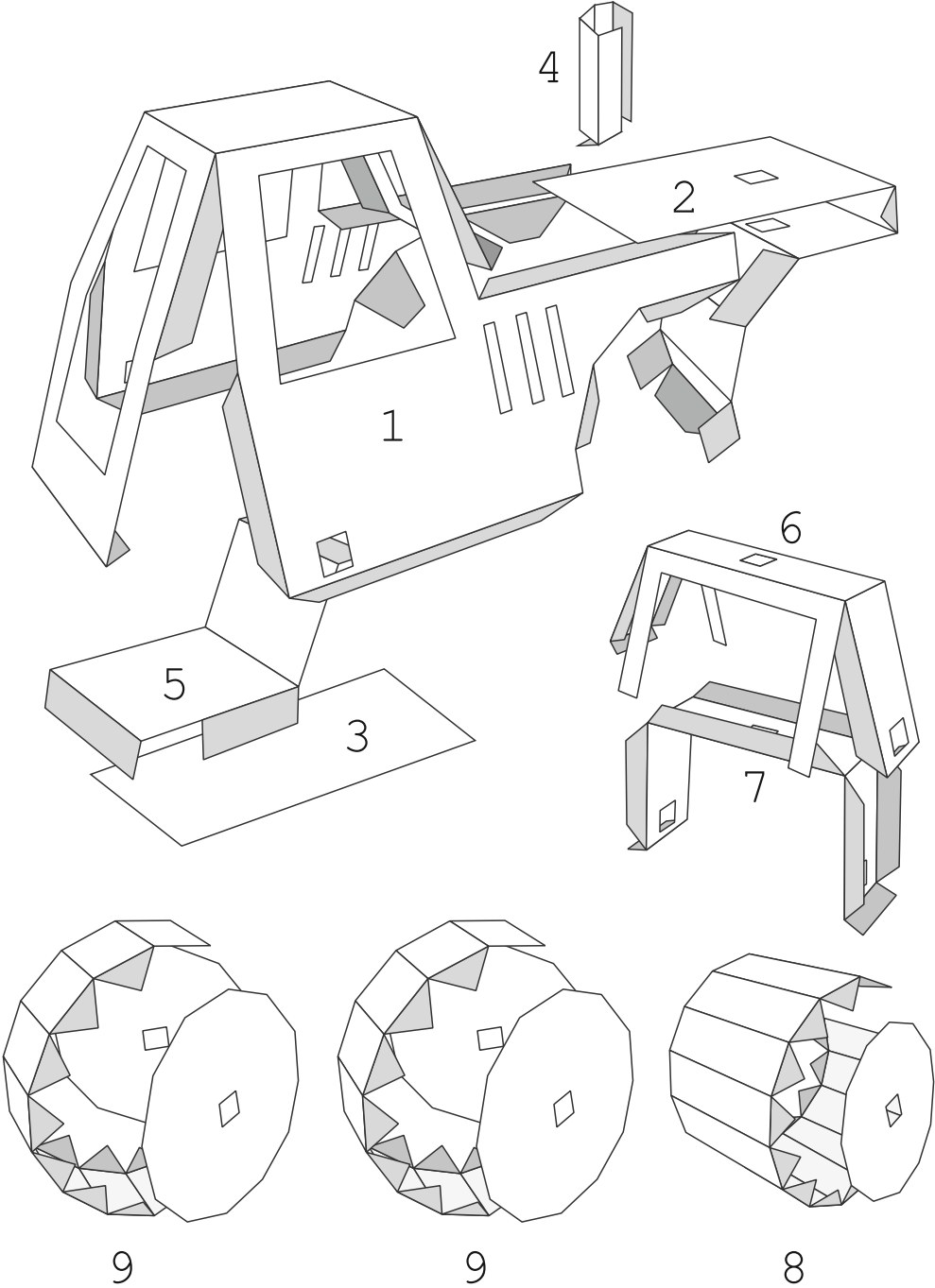
schiacciasassi 2 (esploso)
